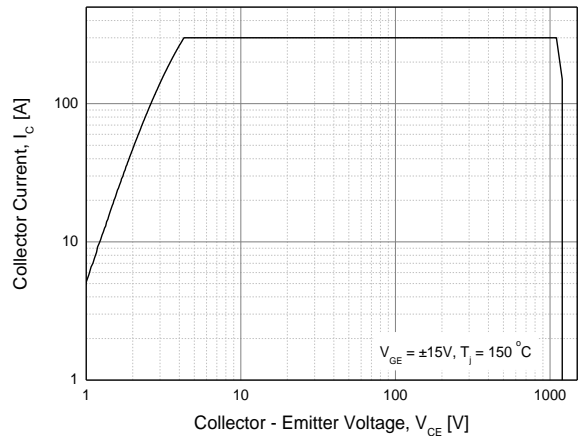
Fig. 12 RBSOA
